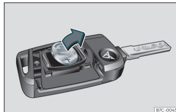
Fig. 73 Llave del vehículo: extracción de la pila.
