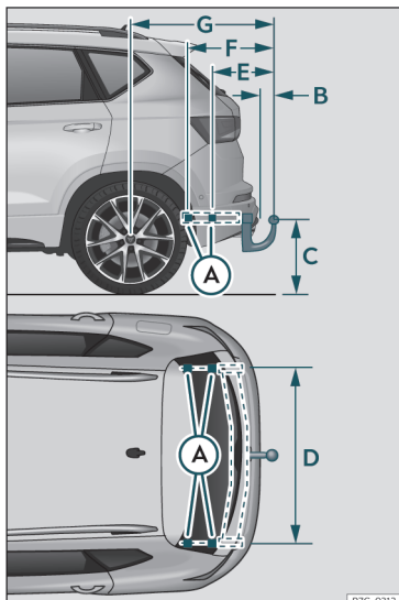
Fig. 196 Cotas y puntos de fijación para el montaje posterior de un dispositivo de remolque.
