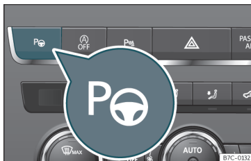
Fig. 177 En la parte superior de la consola central: tecla para conectar el sistema de aparcamiento asistido.
