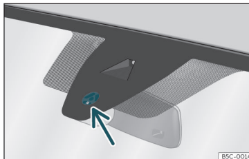
Fig. 130 Sensor de humedad y temperatura del parabrisas.
