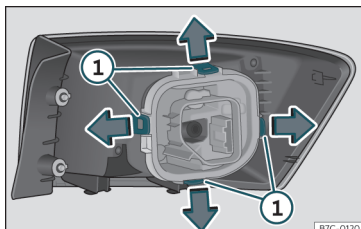
Fig. 50 Lengüetas de fijación en la parte posterior de la unidad de luz trasera.
