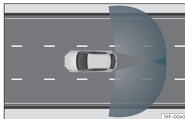
Fig. 152 Zonas de detección de los sensores
