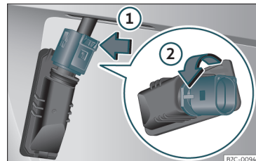
Fig. 54 Luz de matrícula: desmontar el portalámparas.
