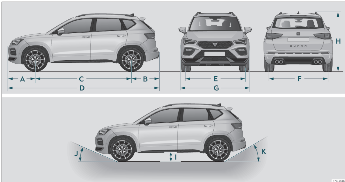
Fig. 215 Dimensiones y ángulos.
