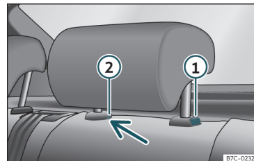
Fig. 105 Apoyacabezas trasero: desmontaje.
