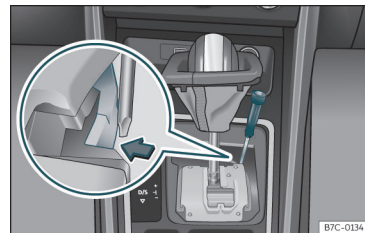
Fig. 145 Palanca selectora: desbloqueo de emergencia en la posición de aparcamiento.
