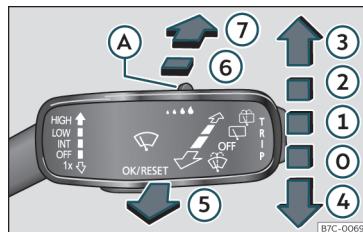
Fig. 96 Manejo del limpiaparabrisas y limpialuneta.
