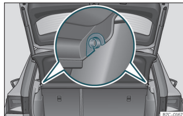
Fig. 111 En el maletero: desmontar y montar la bandeja.
