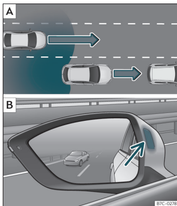
Fig. 172 Representación esquemática: A Situación en un adelantamiento con tráfico en la parte trasera. B Indicación del asistente de cambio de carril en el retrovisor exterior izquierdo.
