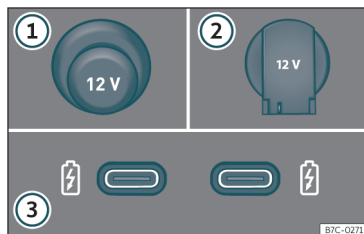
Fig. 127 Tomas de corriente de 12 voltios del vehículo.
