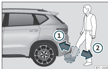
Fig. 85 Portón del maletero con apertura controlada por sensor (Easy Open).
