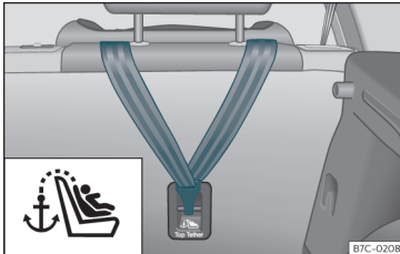
Fig. 28 Parte posterior de los asientos traseros: arrolladoras de sujeción para el cinturón Top Tether.
