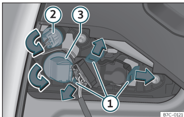
Fig. 52 Desmontar el portalámparas.
