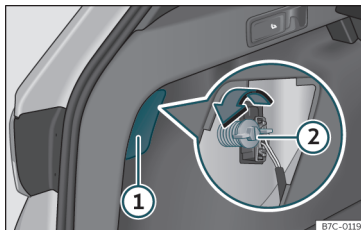
Fig. 49 Maletero: acceso al tornillo de fijación de la unidad de luz trasera.
