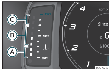
Fig. 61 Indicador de temperatura del líquido refrigerante del motor.
