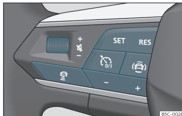
Fig. 161 En el volante multifunción: botones para manejar el ACC
