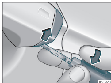
Fig. 79 Manecilla de la puerta del conductor: desprender la tapa haciendo palanca.
