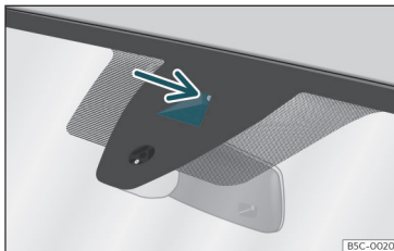
Fig. 150 En el parabrisas: área de campo visual del sistema de aviso de salida del carril.
