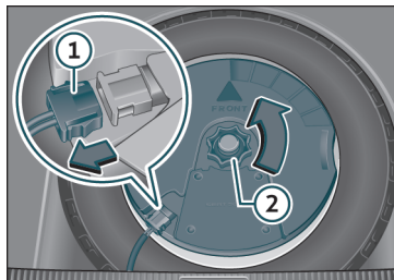
Fig. 214 En el maletero: desmontar el subwoofer.
