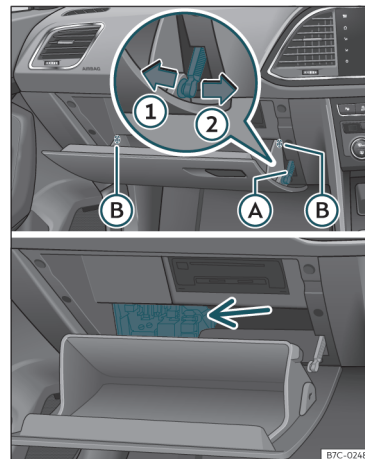
Fig. 46 Guantero (volante a la derecha): acceso a la caja de fusibles.
