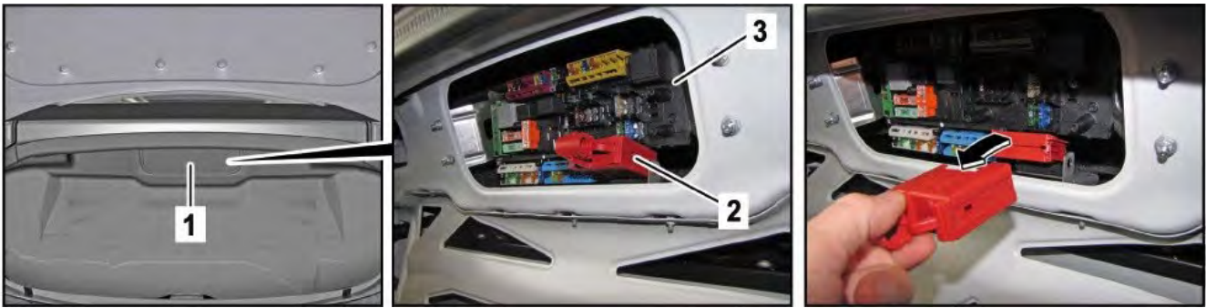
Abrir tapa cobertera (1) / extraer interruptor (2) en la caja de fusibles y relés (3)
